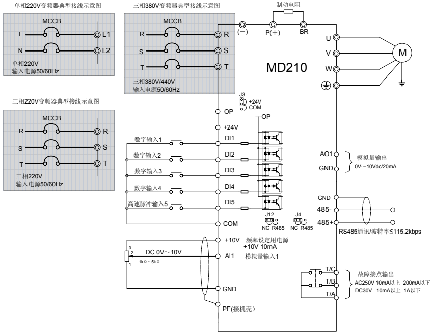
图 3-9 MD210 变频器典型接线示意图
