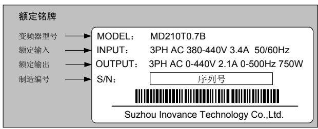
图 2-2 MD210 系列变频器铭牌
