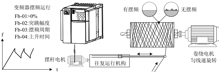
图 4-19 摆频工作模式
