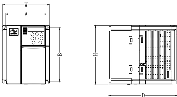
图 2-5 MD210 系列外型尺寸及安装尺寸示意图
