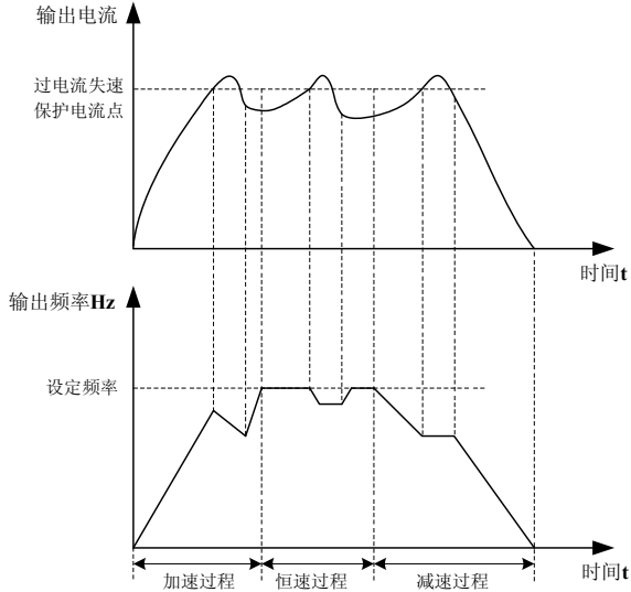
图 6-22 过流失速保护示意图
