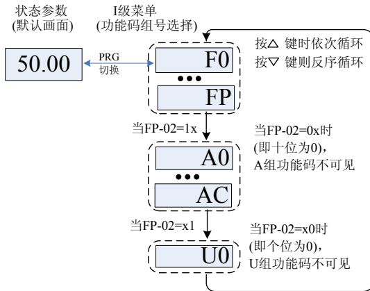
图 4-4 功能码组号浏览操作
