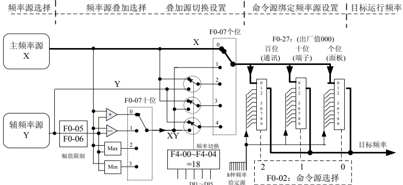
图 4-17 主辅助频率混合给定来源选择
