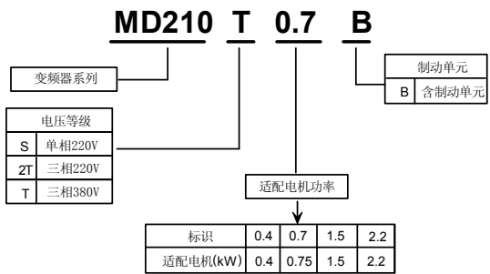
图 2-1 命名规则
