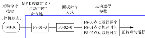
图 4-13 操作面板点动运行
