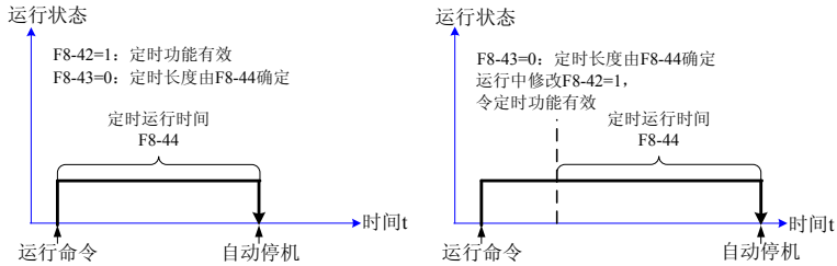
图 4-11 定时停机功能
