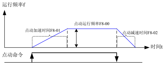
图 4-12 点动运行方式
