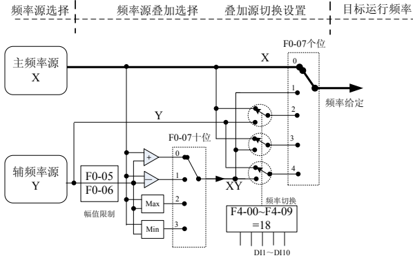
图 6-1 频率源叠加选择示意图
