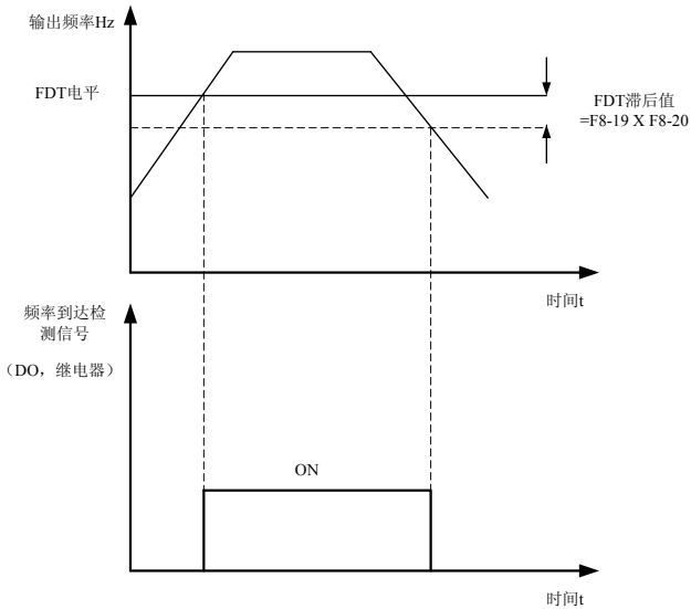
图 6-15 FDT 电平示意图
