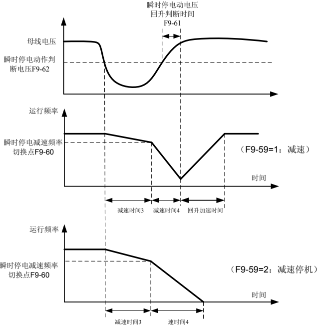
图 6-23 瞬时停电动作示意图
