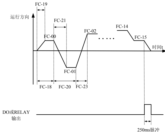
图 6-29 简易 PLC 示意图
