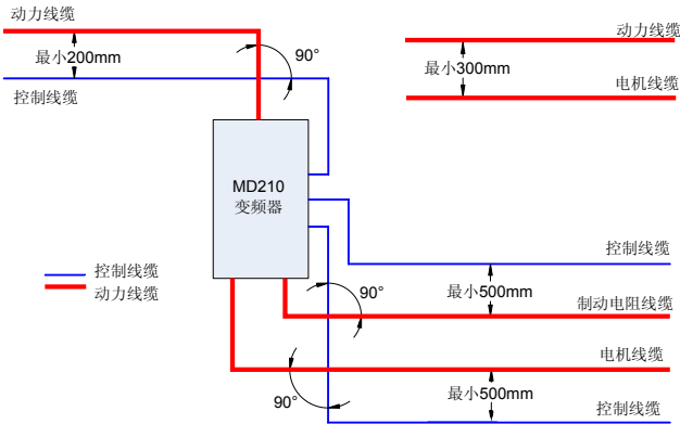
图 7-4 电缆布线图
