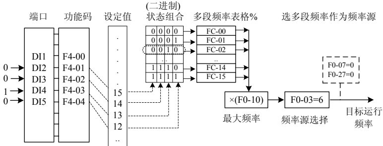
图 4-20 多段速模式的设置
