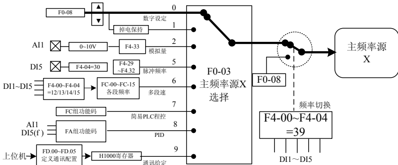
图 4-15 主频率给定来源选择
