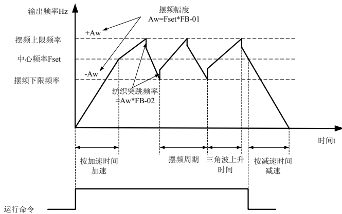
图 6-27 摆频工作示意图
