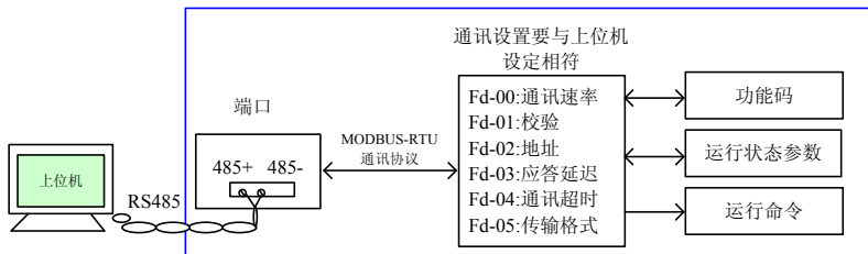
图 4-23 串行通讯设置
