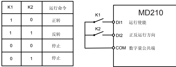
图 6-6 两线式模式 2
