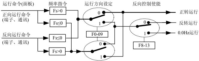
图 4-21 电机运转方向设置
