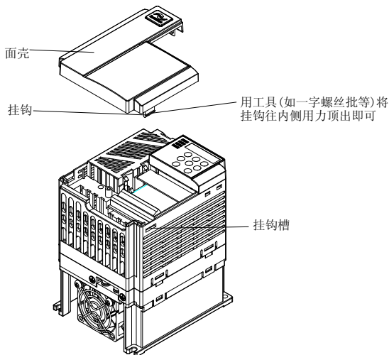
图 3-3 塑胶外壳上盖板拆卸图
