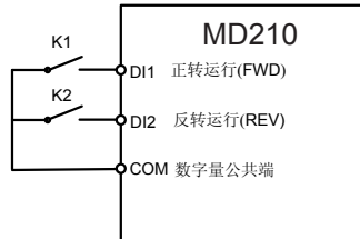
图 6-5 两线式模式 1
