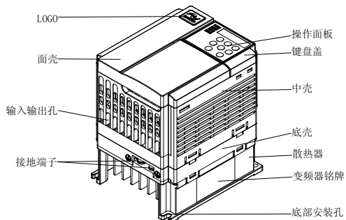
图 2-3 0.4kW-0.75kW 外形图
