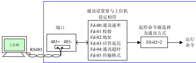
图 4-7 通讯启停控制方式举例
