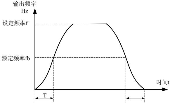
图 6-11 S 曲线加减速 B 示意图
