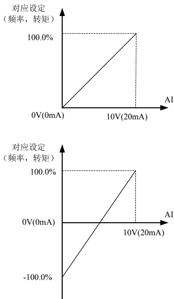
图 6-9 模拟给定与设定量的对应关系
