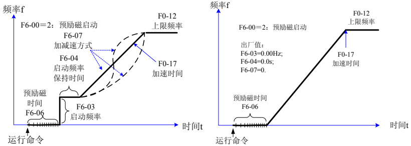
图 4-9 速度跟踪再启动方式
