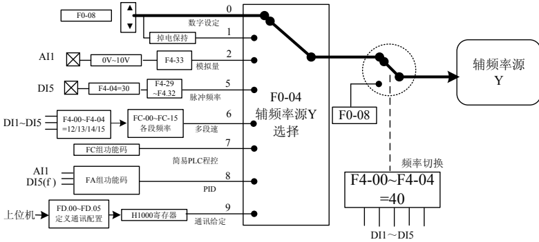
图 4-16 辅助频率给定来源选择
