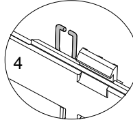
图 7-5 安规电容跳线位置及断开方法
