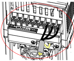
图 7-3 屏蔽电缆接地示意图
