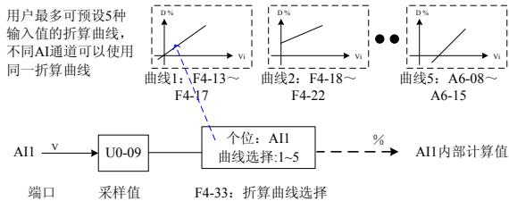
图 4-22 AI 输入信号处理
