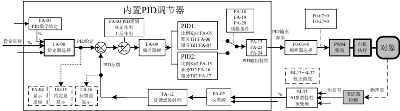
图 4-18 过程控制的频率闭环控制
