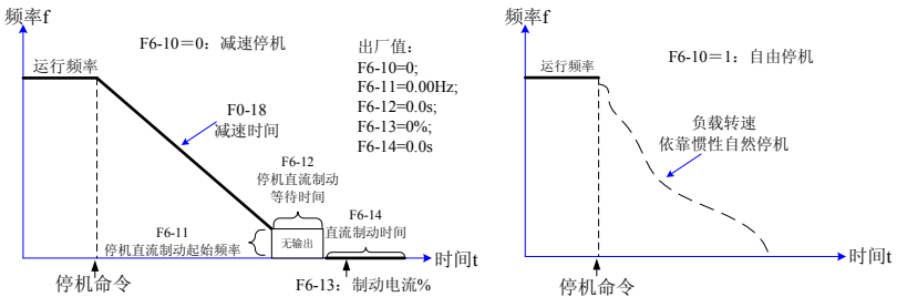
图 4-10 停机模式
