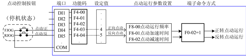
图 4-14 通讯 DI 端口点动运行
